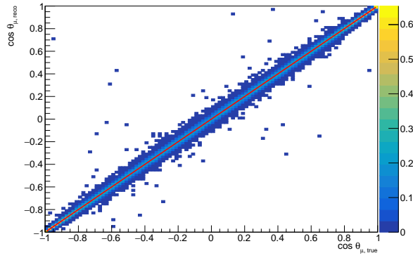
(d) Antimuons
